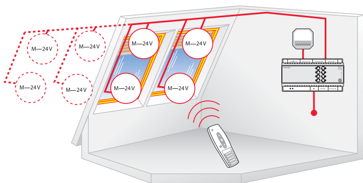
МНОГОКАНАЛЬНЫЙ БЛОК УПРАВЛЕНИЯ VCM 1004 для монтажа в РАСПРЕДЕЛИТЕЛЬНОМ ШИТКЕ.
